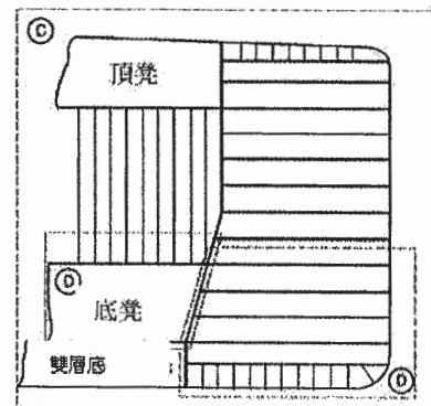
礦砂/油船： 典型橫艙壁
