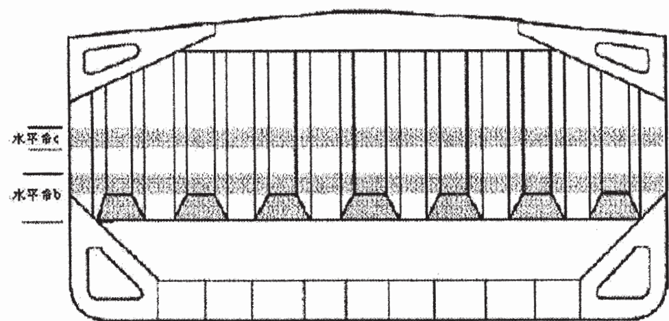
圖2 - 有底艚的船舶
