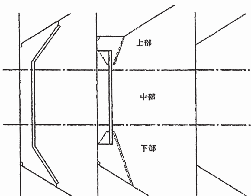
貨艙內典型橫向肋骨 測厚區域Ⓐ
