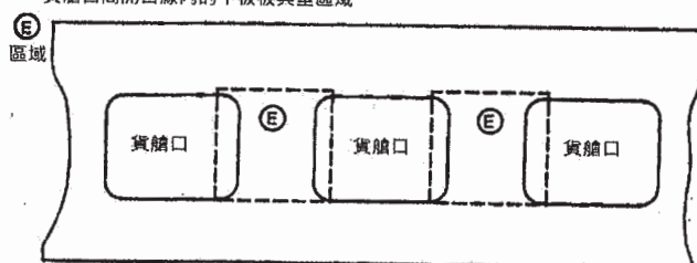
貨艙口間開口線內的甲板板典型區域
