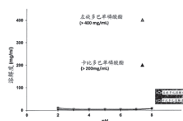
左旋多巴L-多巴羧酸和卡比多巴L-多巴羧酸的溶解度
